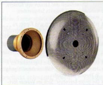
■ Neue „FitStar“-Ansaugungen aus dem Hause Hugo Lahme nach DIN 13 451; Foto: Hugo Lahme, Ennepetal
